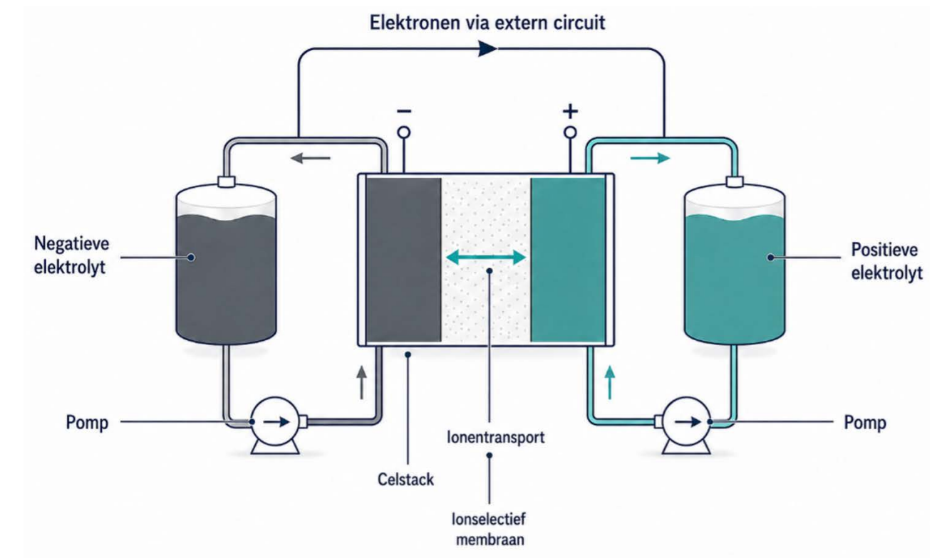
Figuur B1.3 Principe van een flowcelbatterij met externe elektrolyttanks, pompen en een elektrochemische celfiguur
