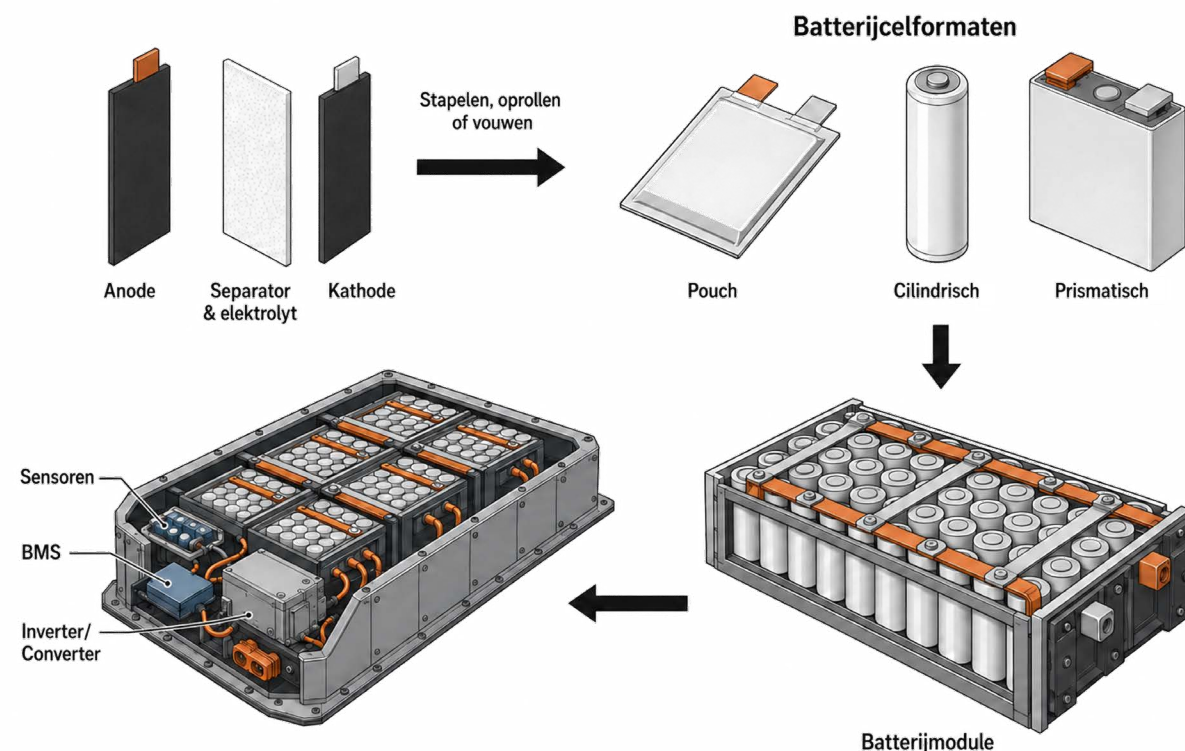
Figuur 4 Schematische weergave van batterijcomponenten, cellen, modules, accupakketten en systemen
