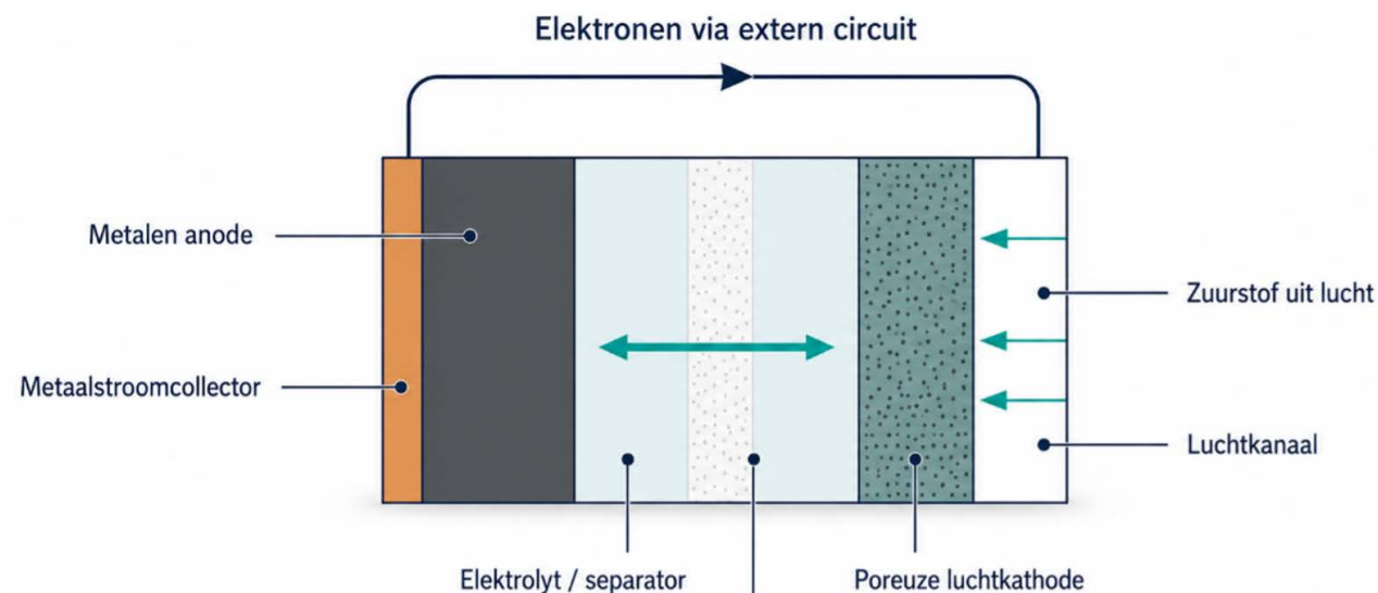
Figuur B1.4 Principe van een metaal-luchtbatterij, waarbij reversibele oxidatie van de poreuze luchtkathode een onderdeel is van de batterijwerking
