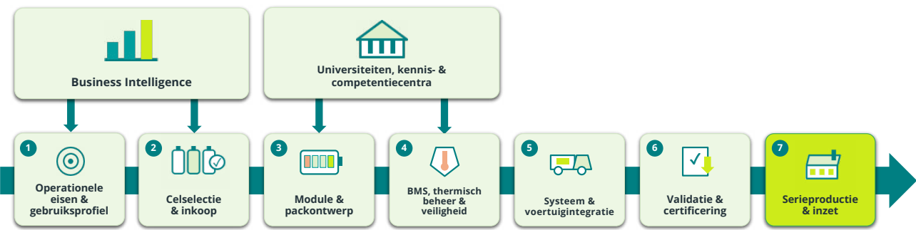
Figuur 6 Het scala aan activiteiten dat komt kijken bij het ontwerpen, integreren en opschalen van een heavy-duty en dual-use batterijsysteem: van BI en operationele eisen tot celselectie, module- en packontwerp, BMS en thermisch beheer, systeemintegratie, validatie en certificering, en uiteindelijk serieproductie en uitrol
